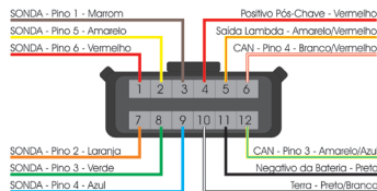
Vista Traseira do Conector do Chicote
