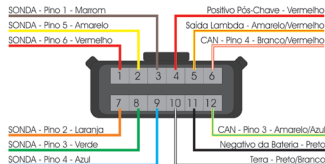
Vista Traseira do Conector do Chicote
